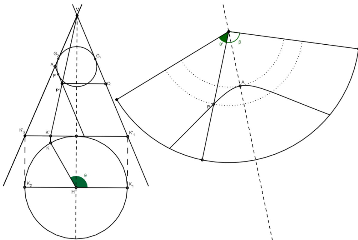
Figura 3: Proiezioni ortogonali della costruzione di Dandelin sul piano \beta e sul piano \tau e sviluppo del cono nel caso della parabola.
