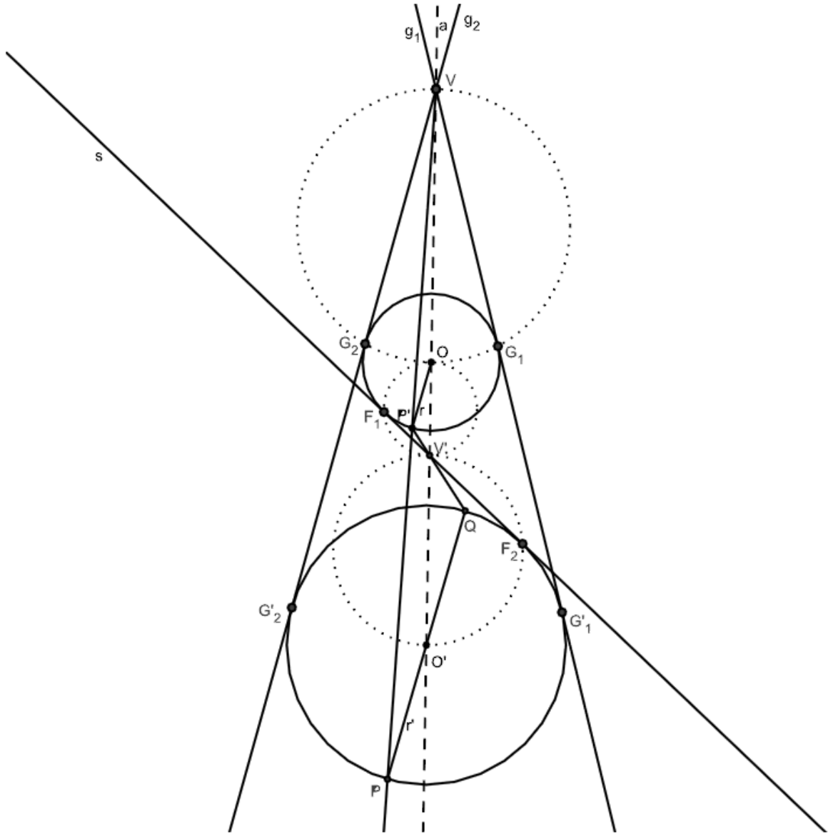
Figura 1: Sezione della costruzione di Dandelin con il piano \beta .
