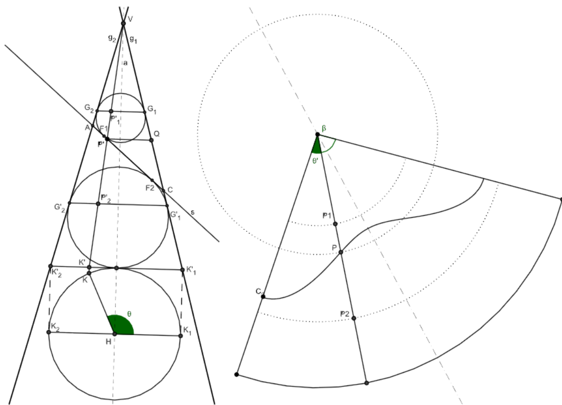
Figura 2: Proiezioni ortogonali della costruzione di Dandelin sul piano \beta e sul piano \tau e sviluppo del cono.
